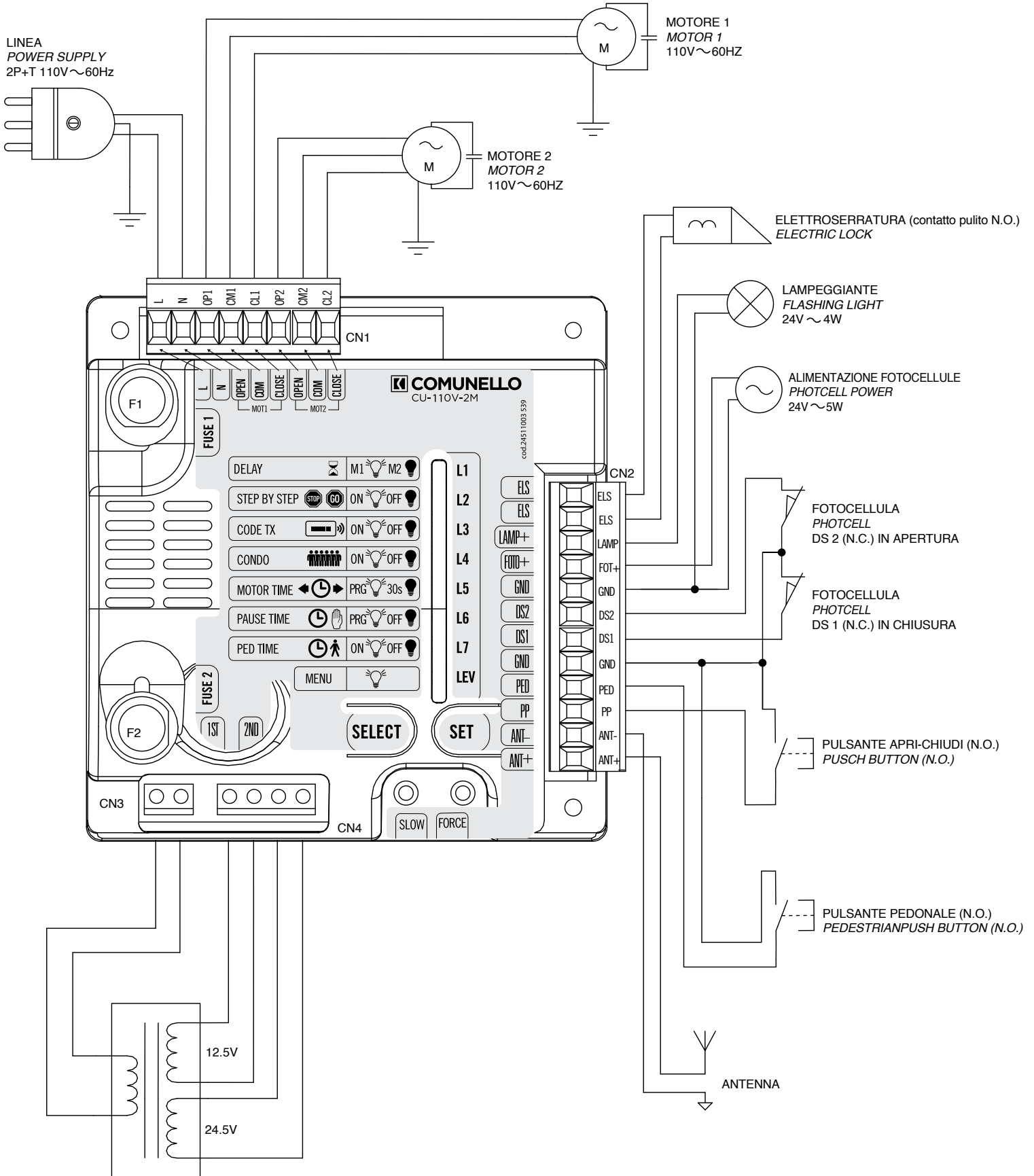
TRASFORMATORE TRANSFORMER 230 / 24.5V - 0.4A; 12.5V - 0.17A
